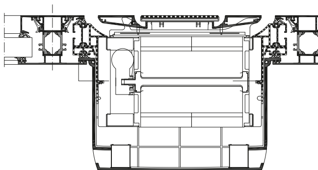
Вариант монтажа AWS 60 вровень изнутри Installation example of AWS 60, flush-fitted on the inside
