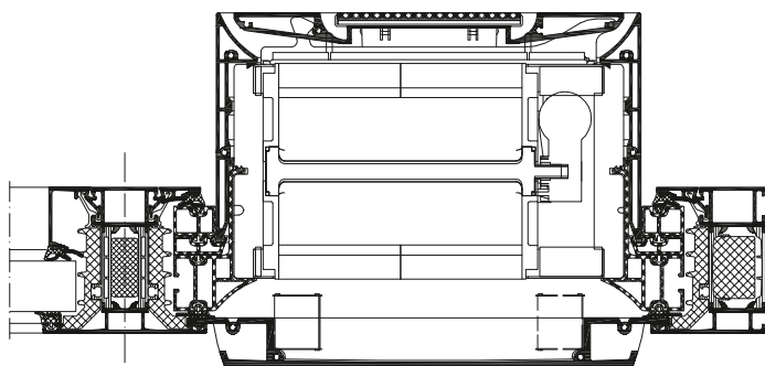
Вариант монтажа AWS 75.SI+ вровень снаружи Installation example of AWS 75.SI+, flush-fitted on the outside
